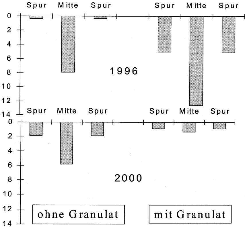
Abbildung 2: Luftleitfähigkeit im Oberboden (0-10 cm) Oberboden (0-10 cm)
